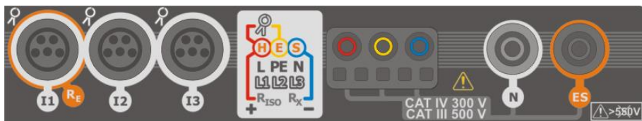
Rys. 5.1 Wejścia pomiarowe
